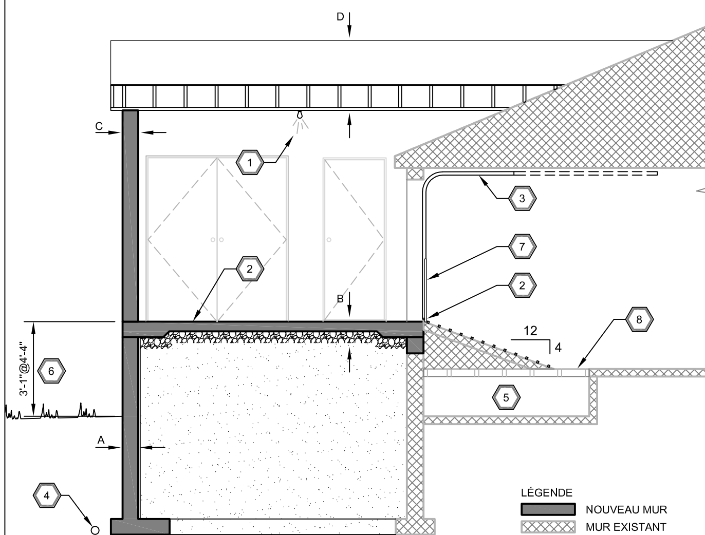
COUPE QUAI 2 SORTIE À 90°
