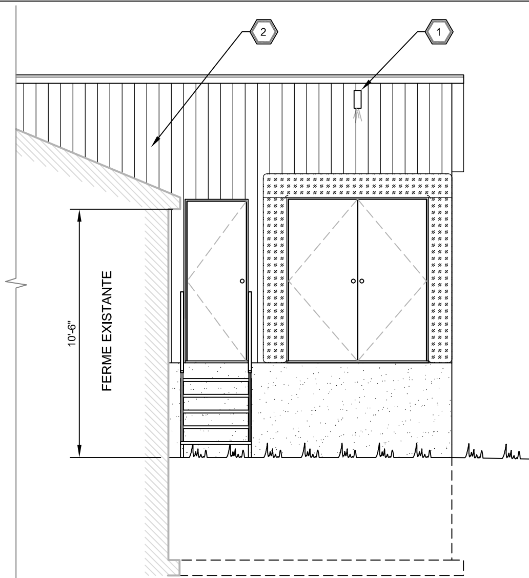
ÉLÉVATION DE GAUCHE
