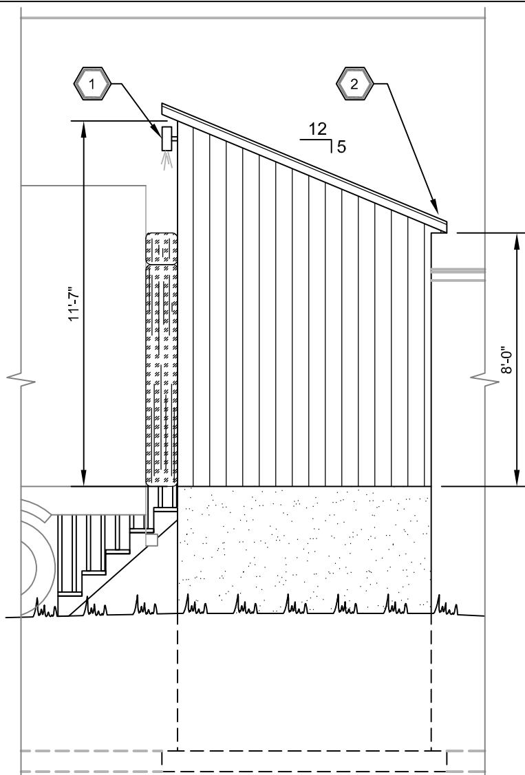
ÉLÉVATION DE FAÇADE
